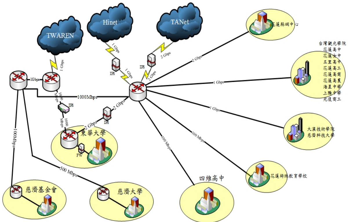
圖 2.6 花蓮區網中心網路連線架構圖
